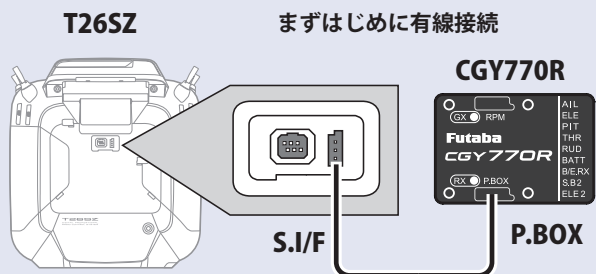
CGY 接続コード (ジャイロに付属)
